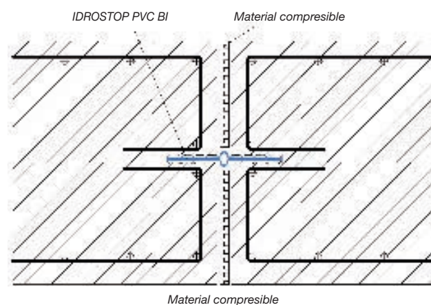
Esquema del posicionamiento del Idrostop PVC BI
